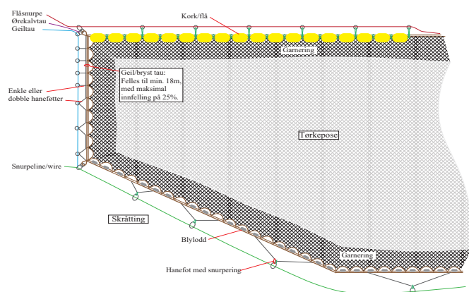
Figur 1: Rigging av geila slik det ble foreslått under Gardermoemøtet. Notas lengde i brystenden skulle begrenses av et geil-tau på minimum 18 m og en maksimal innfelling langs geil-tauet på 25 %.
