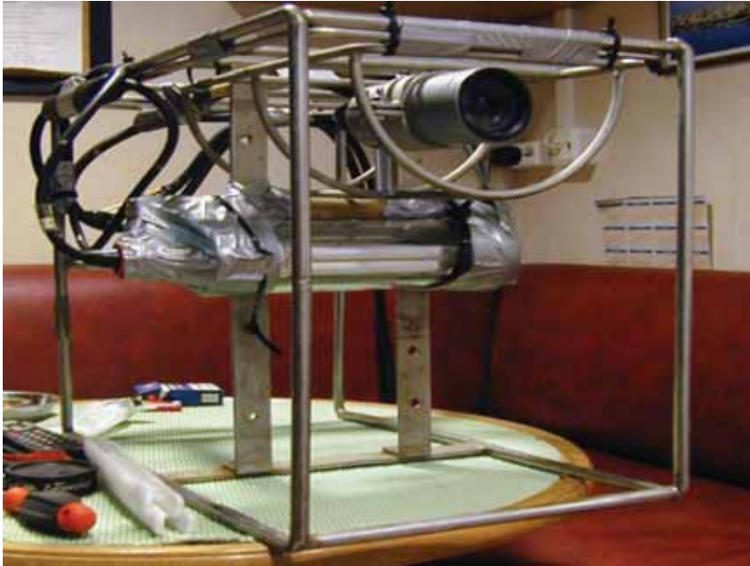
Figur 2. Kamera rigg med CCD-kamera og lysutstyr for dyp ned til 500 meter.
