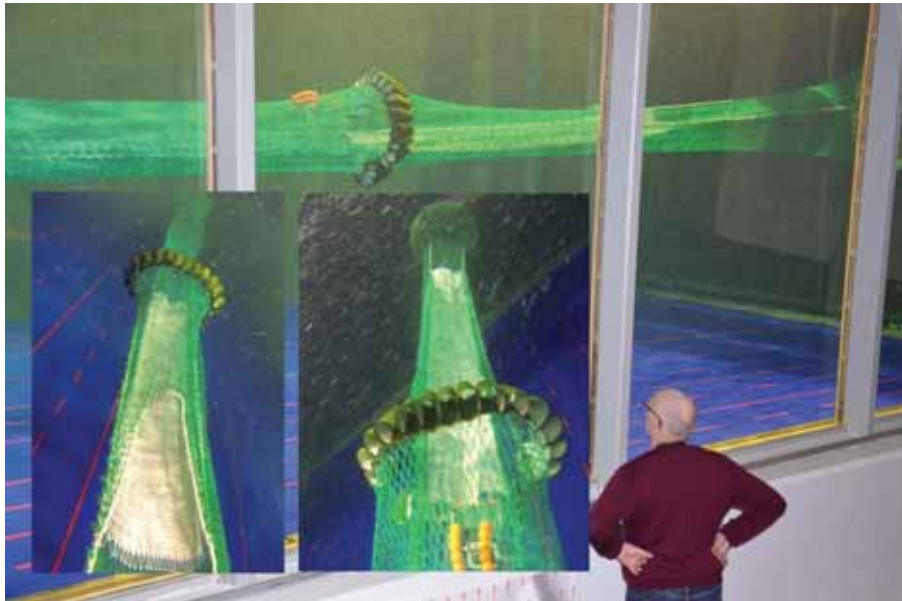
Bilde 14. Forlengelse utspilt med kites. På det innfelte bildet til venstre ser vi utslippshullet bakfra.
