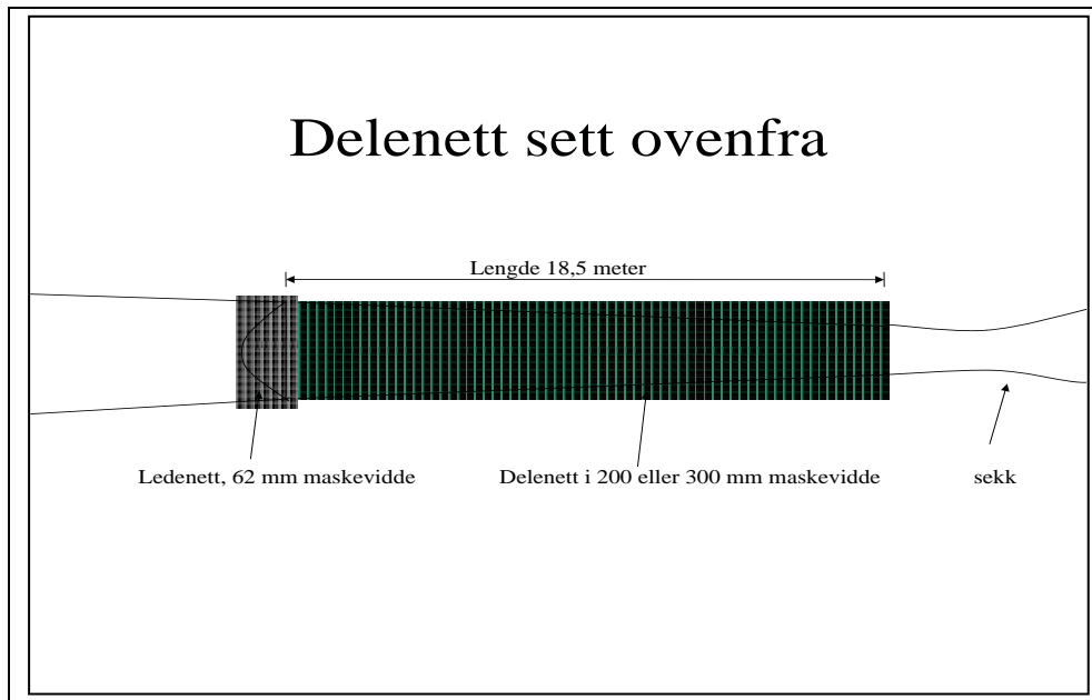
Figur 1. Skillepanel sett ovenfra med ledeneett, og delenett.
