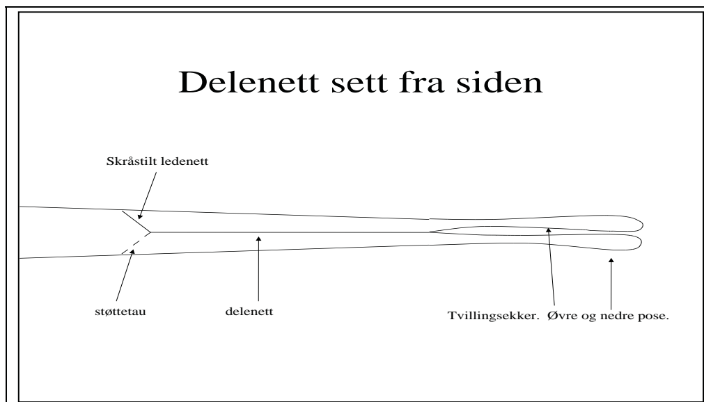
Figur 2. Skillepanel sett fra siden med ledeneett, delenett og tvillingposer, et oppsett som ble benyttet under forsøkene for å undersøke fangstfordelingen av torsk og hyse over og under nettet
