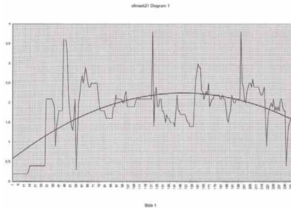
Figur 5. Diametermålinger med Scanmar avstandsmålere i området med ca 250 masker total omkrets i vanlig sylinder uten nett. Diameter synes størst omlag midt halet.
