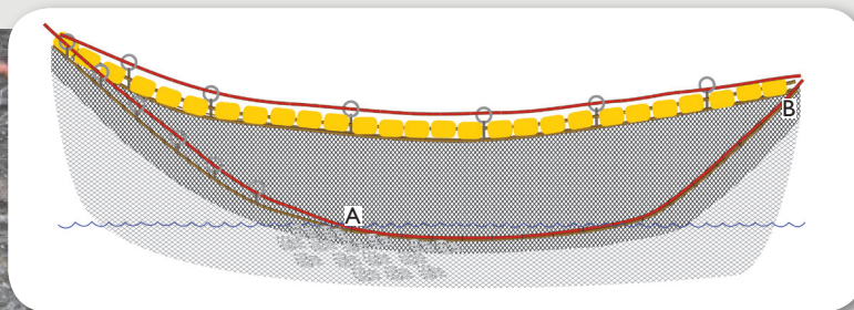
Figur 4: Omarbeidet flåsnurpe. Flåsnurpa er bendslet fast i avlastningstelna mellom punktene A og B. Ca. 1/3 av den nye flåsnurpa går fortsatt gjennom ringene.
