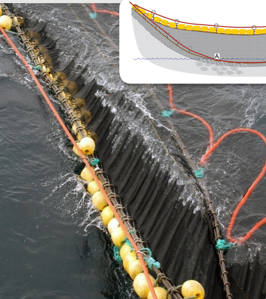
Figur 4: Omarbeidet flåsnurpe. Flåsnurpa er bendslet fast i avlastningstelna mellom punktene A og B. Ca. 1/3 av den nye flåsnurpa går fortsatt gjennom ringene.
